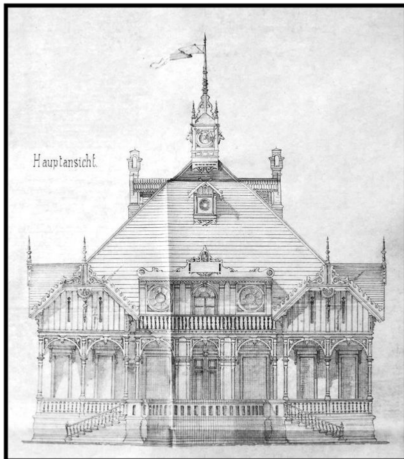
Projekt leśniczówki w Lipniku, Emanuel Rost sen.
